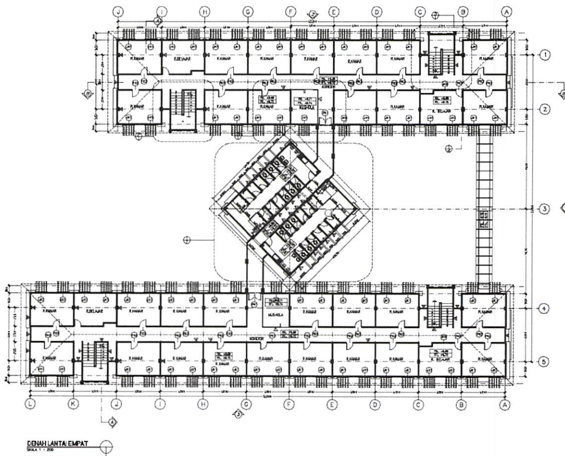
Gambar 2. Denah Lantai 4 dan Pola Atap Gedung D
